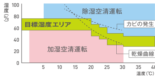
■ おまかせ運転開始時の運転モード
