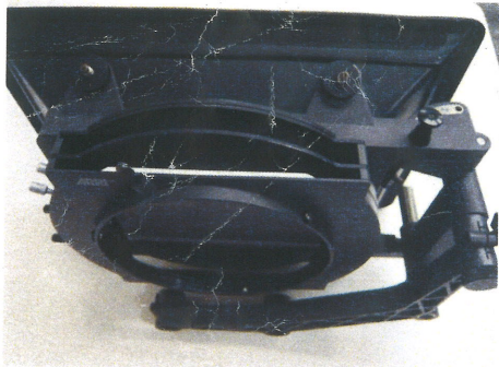
MB-14 19mm Rods 6.6" × 6.6" プロダクションマットボックス 3 フィルターステージ
