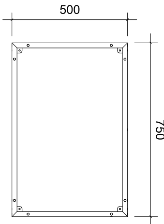
正面フレーム (A-500) P-2 front view
