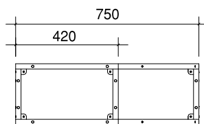
上面フレーム P-22 top view
