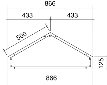
正面フレーム P-49 front view
