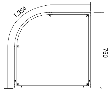
正面フレーム P-21 front view
