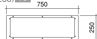
上面フレーム (YD-250/YF-250) P-5 Top view
