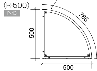
側面フレーム side view
