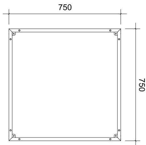
正面フレーム (A) P-1 front view
