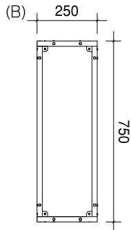
側面フレーム P-3 side view
