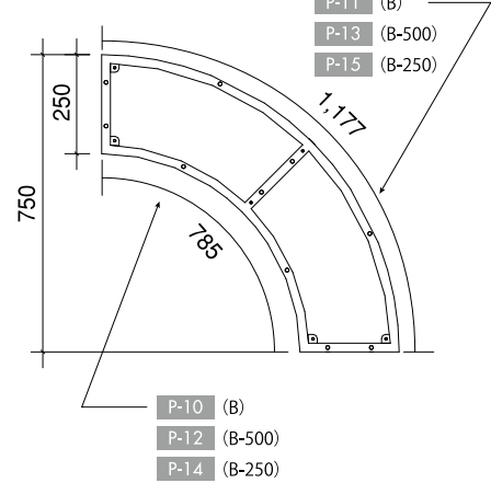
上面フレーム (B/B-250/B-500) P-9 top view
