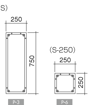
側面フレーム side view
