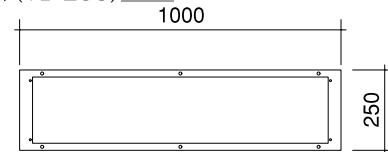
底面フレーム (YF-250) P-3 bottom view
