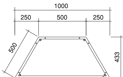
正面フレーム (YD-250) P-55 front view
