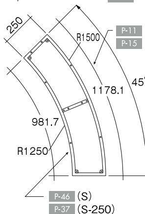
上面フレーム (S/S-250) top view
