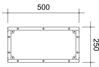
上面フレーム (A-500) P-5 top view
